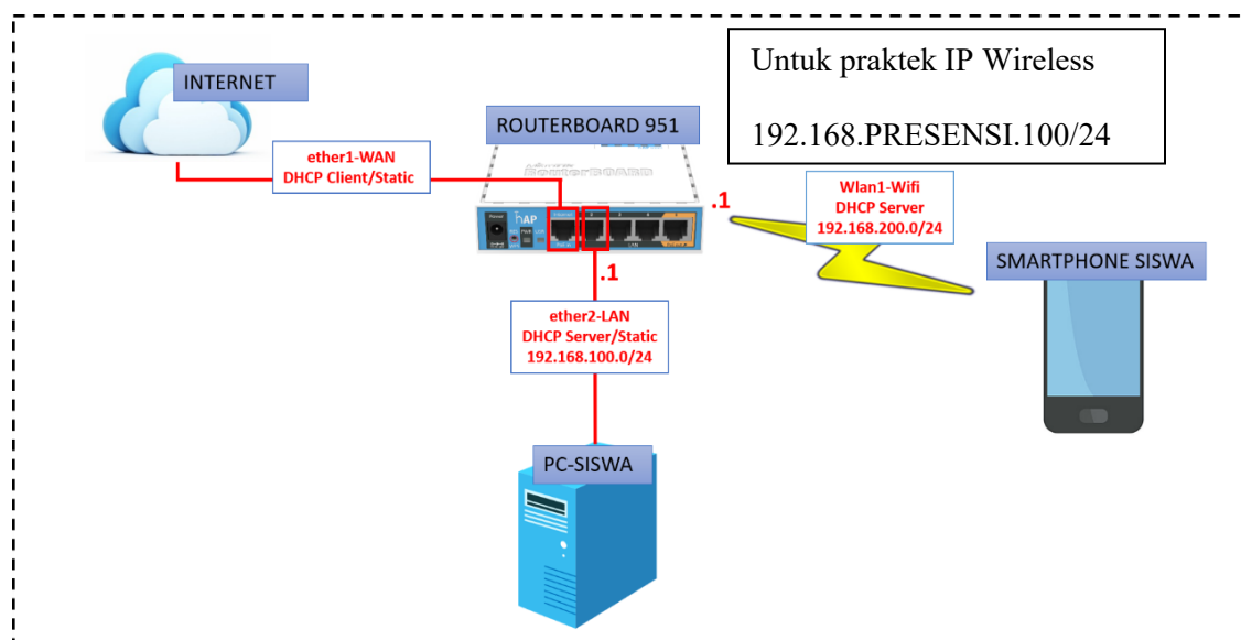
Gambar 1.1 Topologi Jaringan
