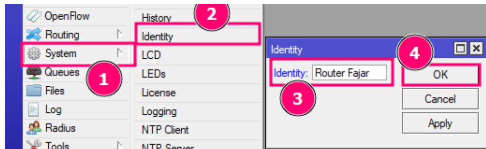
Gambar 1.5 Merubah Identitas
