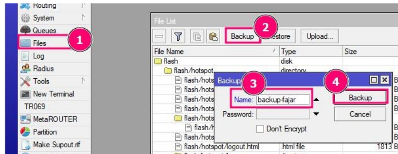
Gambar 1.16 Backup Konfigurasi
