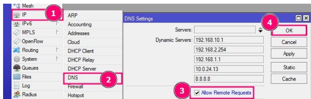
Gambar 1.10 Konfigurasi DNS
