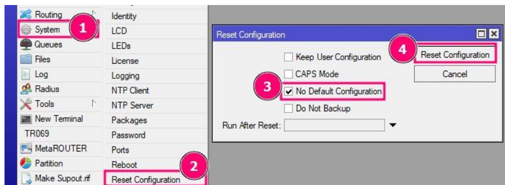
Gambar 1.4 Reset Mikrotik
